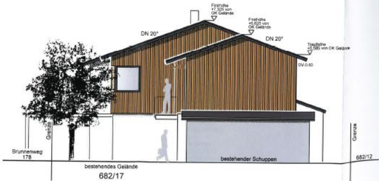
ANSICHT OST (NEUER ZUSTAND)
